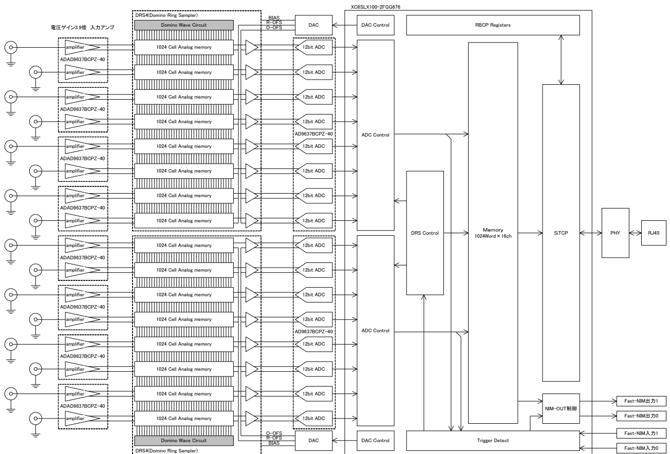
図 4-1 16ch-1Gsp/s-Digitizer・ブロック図
